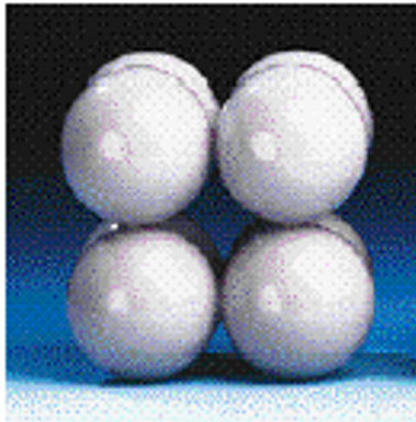
simple cubic
